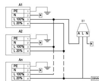
Схема подключения светильников ФОТОН-ОФИС ( ФОТОН-ПРОМ ) с возможностью ступенчатого диммирования
